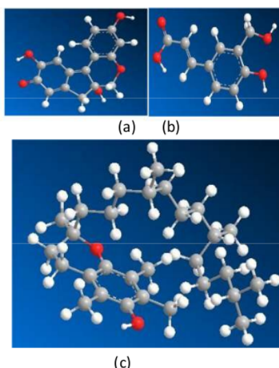
mol2 {SYBYL2(*.mol2)} (Gbr. 3).
