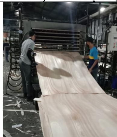
Proses Kerja di Unit Hot Press Plywood
